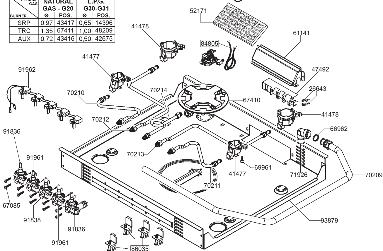
NOZZLES TABLE
