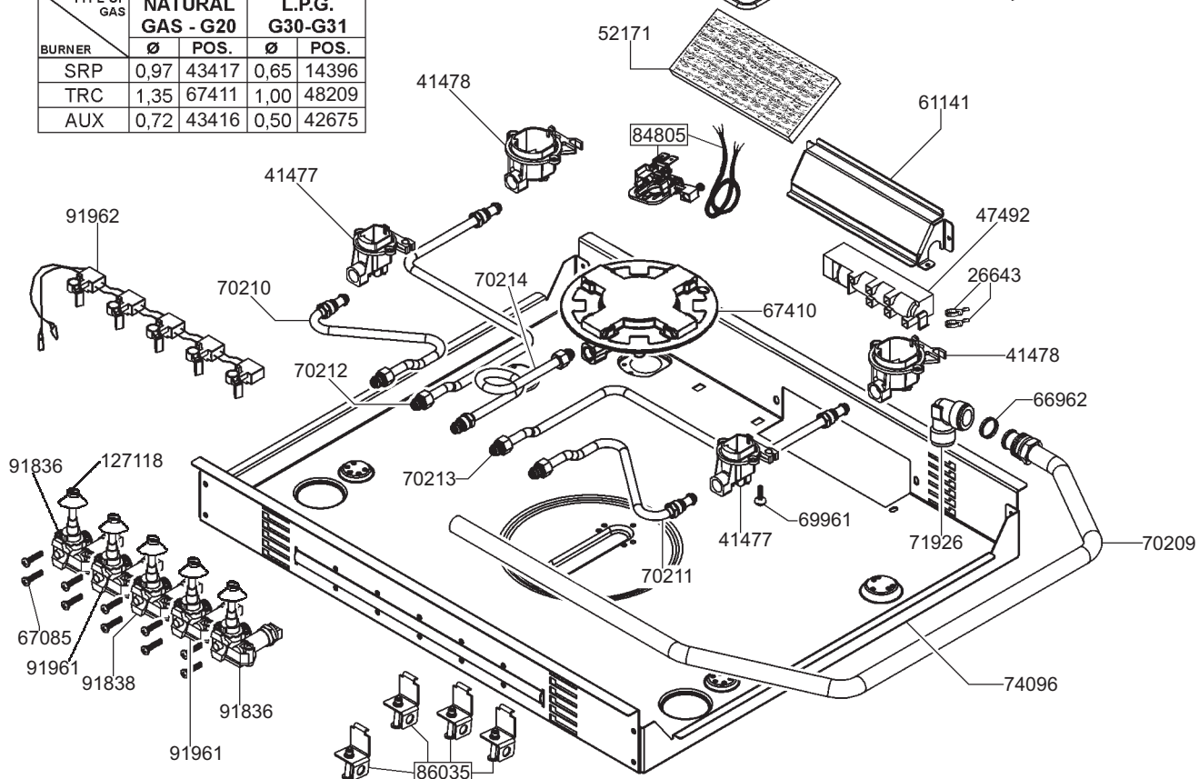
NOZZLES TABLE
